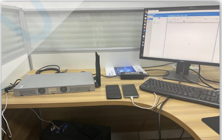
商用手机终端+ USRP-LW N321模拟基站
