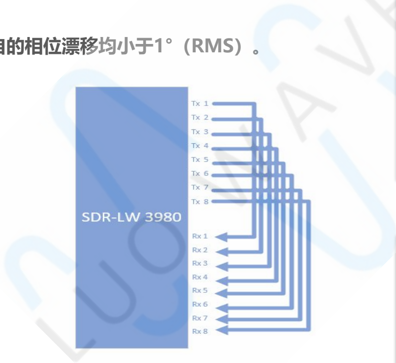
通道间相位差测试连接图
